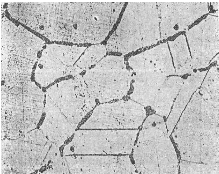
Промежуточная структура (500 X )
