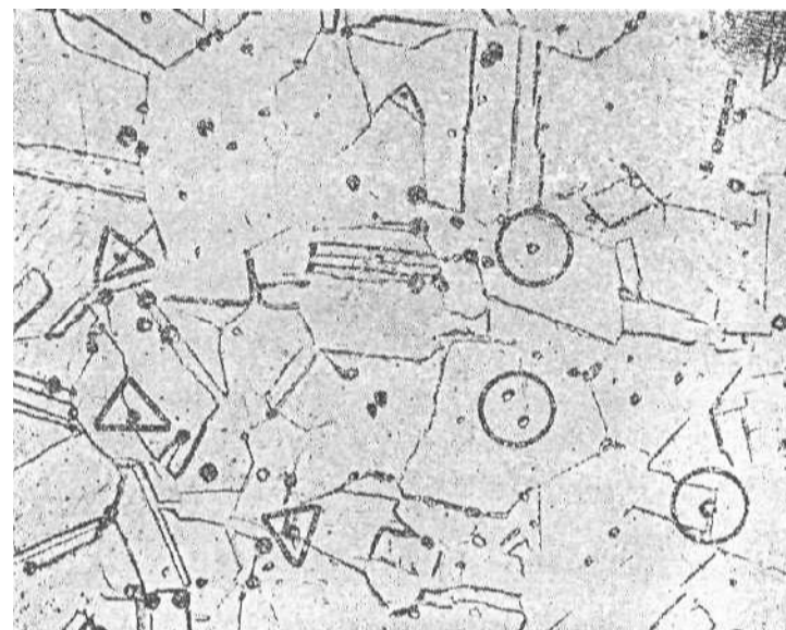
Зернограничный пitting I (500 X )
