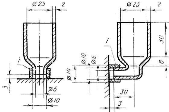
а — сосуд для испытаний горизонтальных поверхностей; б — сосуд для испытаний вертикальных поверхностей; 1 — резиновая манжета Черт. 7
