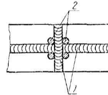
1 — сварной шов; 2 — места анодного травления Черт. 8
